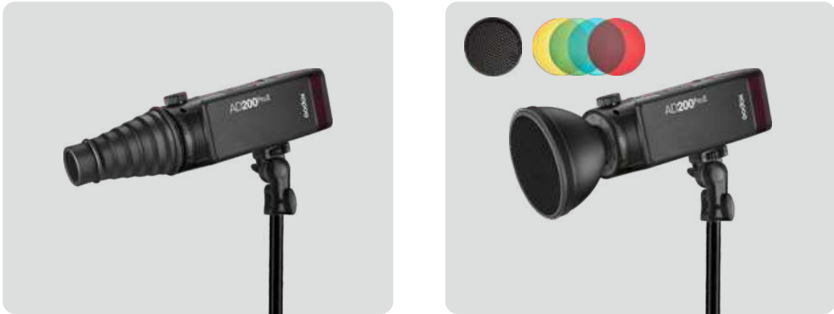
AD-S9 束光筒 适用于H200J裸管灯头 AD-S2+AD-S11 反光罩+蜂巢&色片 适用于H200J裸管灯头
